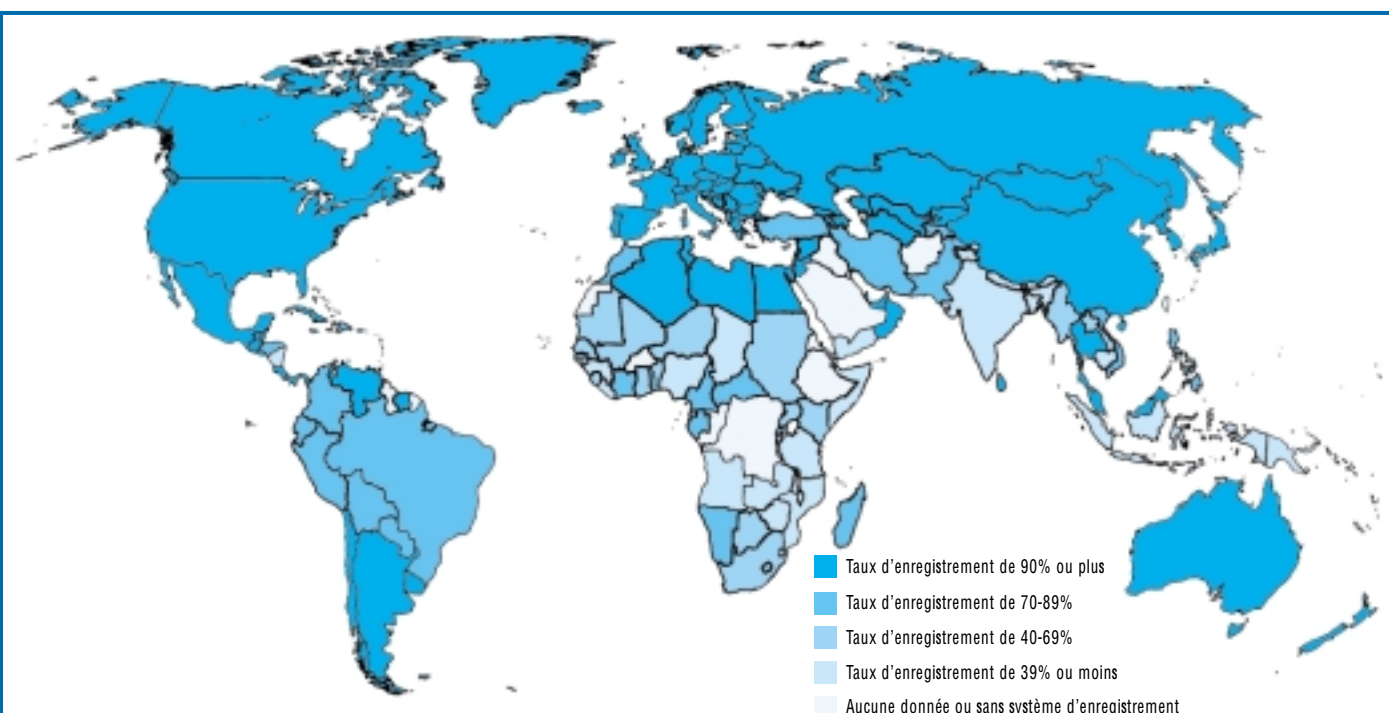
Figure 2 : Niveaux d'enregistrement des naissances, estimations pour 2000
